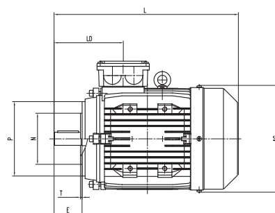
IM B14 (IM 3601)
