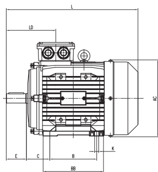
IM B3 (IM 1001)
