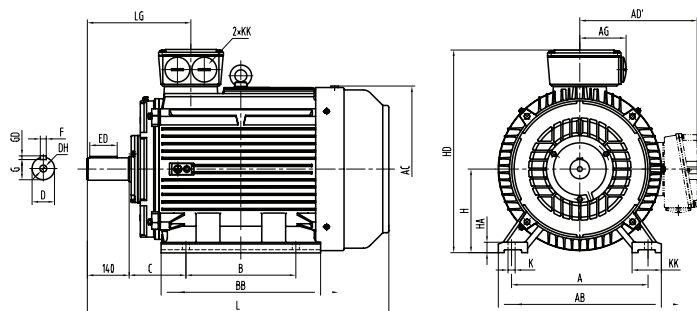
IM B3 (IM 1001)
