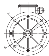
IM B5 (IM 3001) - V1 (IM 3011)
