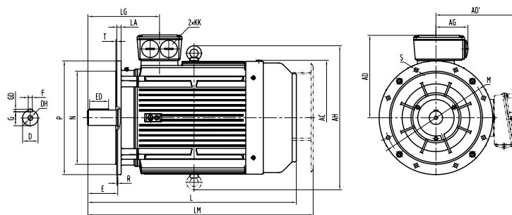
IM B5 (IM 3001) - V1 (IM 3011)
