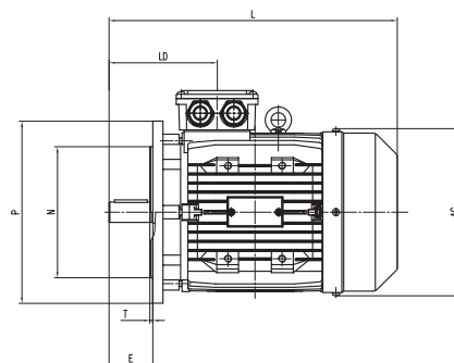
IM B5 (IM 3001) - V1 (IM 3011)
